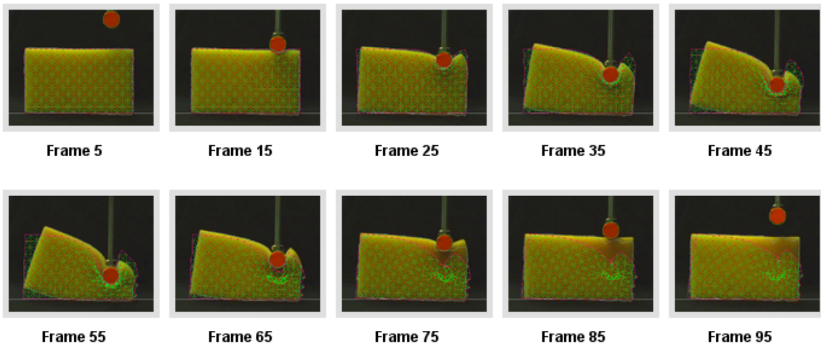
FIGURE 10.12: Test data.
